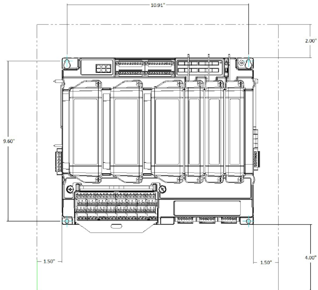
Рисунок А1: Габаритный чертеж и зазор для корпуса .
